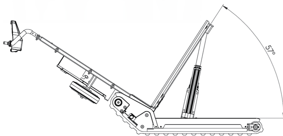
Maximale Neigungsposition Ladefläche
